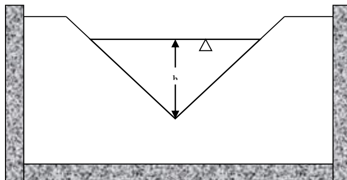
90 ° V-Notch
